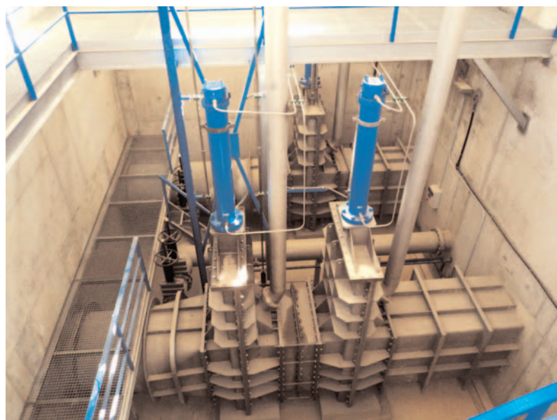
Fig. 7. Caseta de desagüe.
